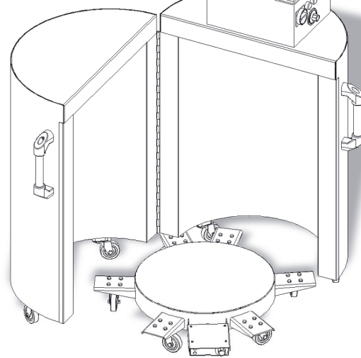
Chauffe-fût électrique avec plaque chauffante mobile.
