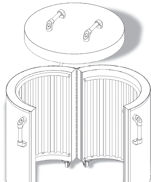
Chauffe-fûts à vapeur avec couvercle isolant séparé. Calentador de barril de vapor con tapa aislante separada.
